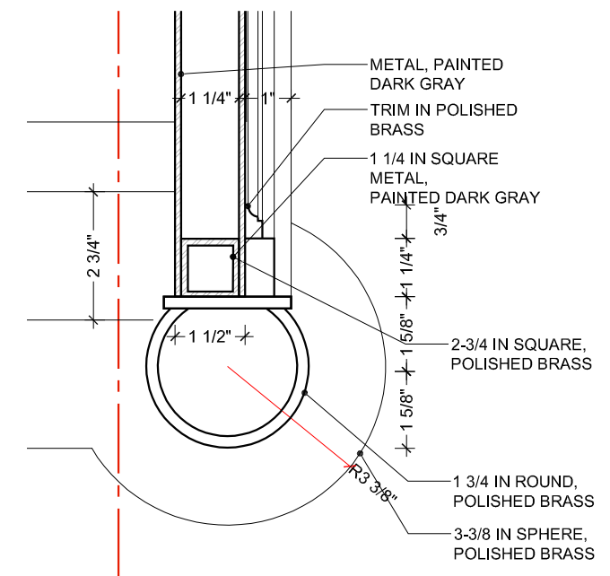
MARQUEE DETAIL - BOTTOM MOLD- ING
