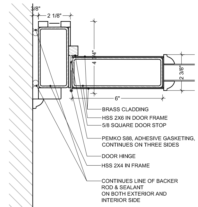
DOOR DETAIL - JAMB
